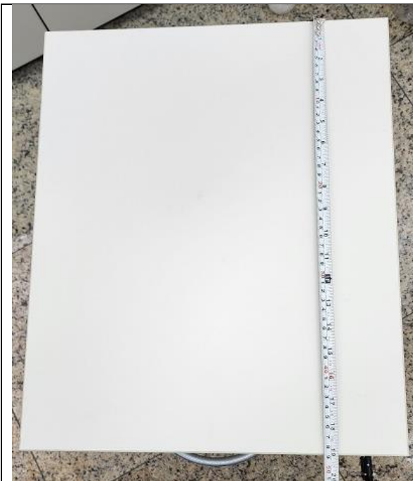
Dimensões: 300(l) x 520(p) x 560(h) mm. Tolerâncias dimensionais: +/- 2%. Profundidade apresentada: 490mm Tolerância: 510-530mm
