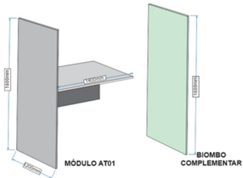
Imagem ilustrativa 1, contendo o módulo e biombo complementar.
