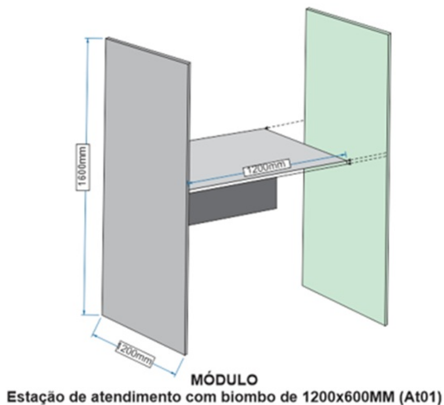
Imagem ilustrativa 5, contendo o módulo e biombo complementar (estação completa – montagem)
