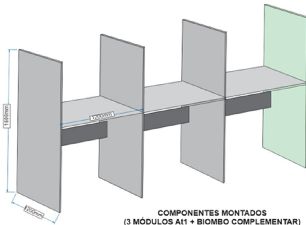
Imagem ilustrativa 6, contendo 3 módulos e biombo complementar
