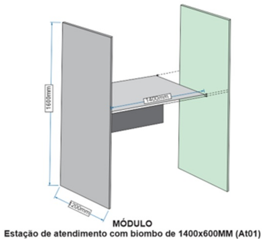
Imagem ilustrativa 2, contendo o módulo e biombo complementar (estação completa – montagem)
